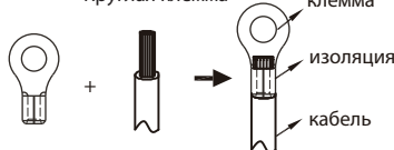
Круглая клемма
